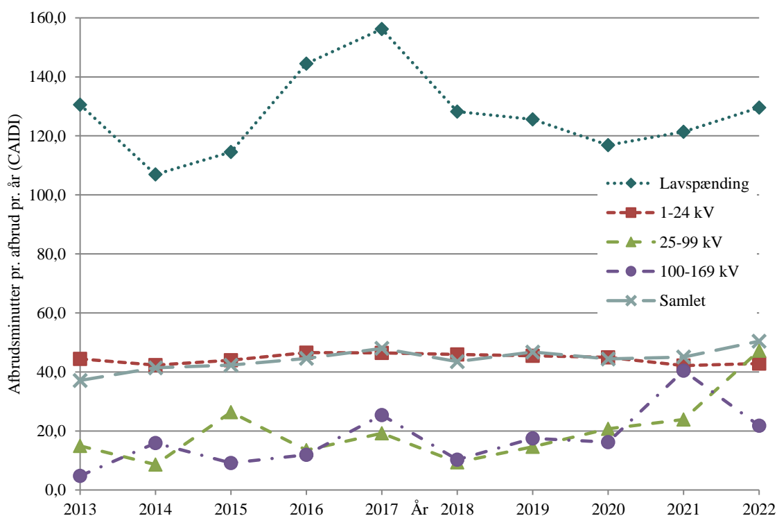
Figur 4.6 Gennemsnitligt antal minutter en kunde er afbrudt opgjort på forskellige statistikområder
