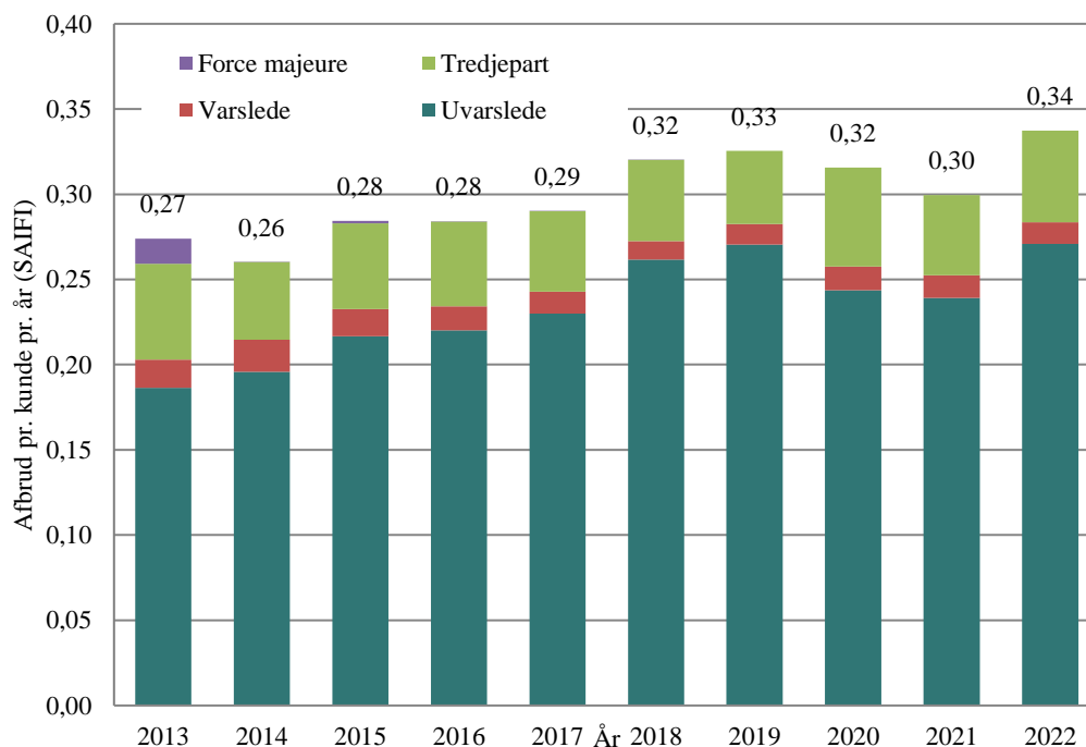
Figur 5.3 Fordelingen af antal gennemsnitlige kundeafbrud opgjort på 1-24-kV-statistikområdet (SAIFI)
