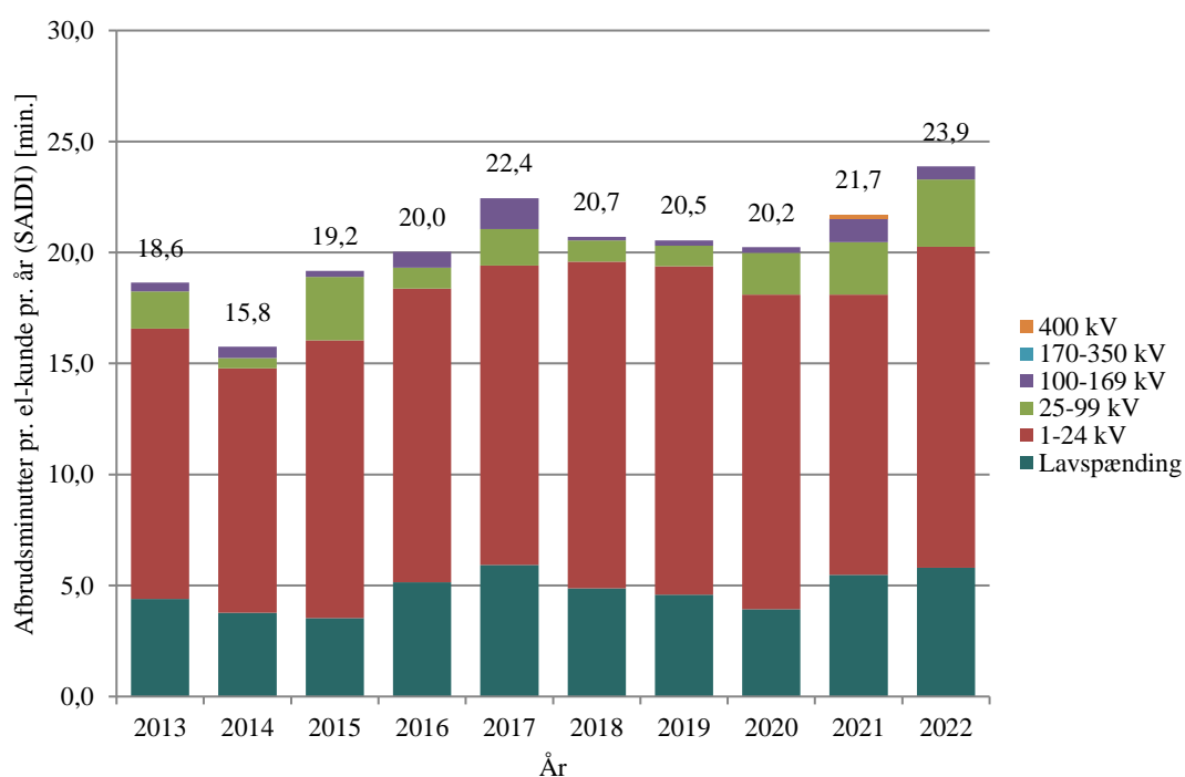
Figur 4.2 Gennemsnitlig afbrudsvarighed pr. kunde i minutter opgjort på statistikområder pr. år (SAIDI)
