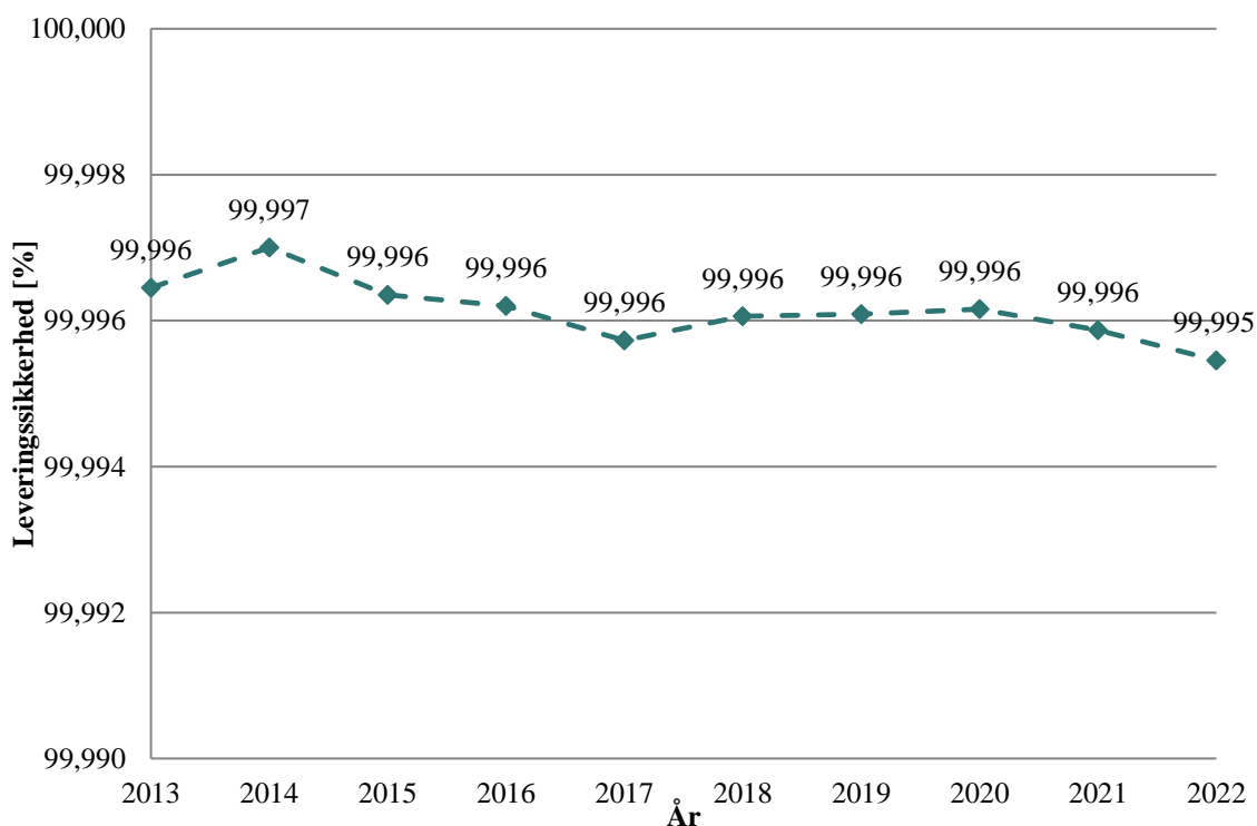
Figur 4.1 Leveringssikkerhed i procent pr. år, ASAI 5
