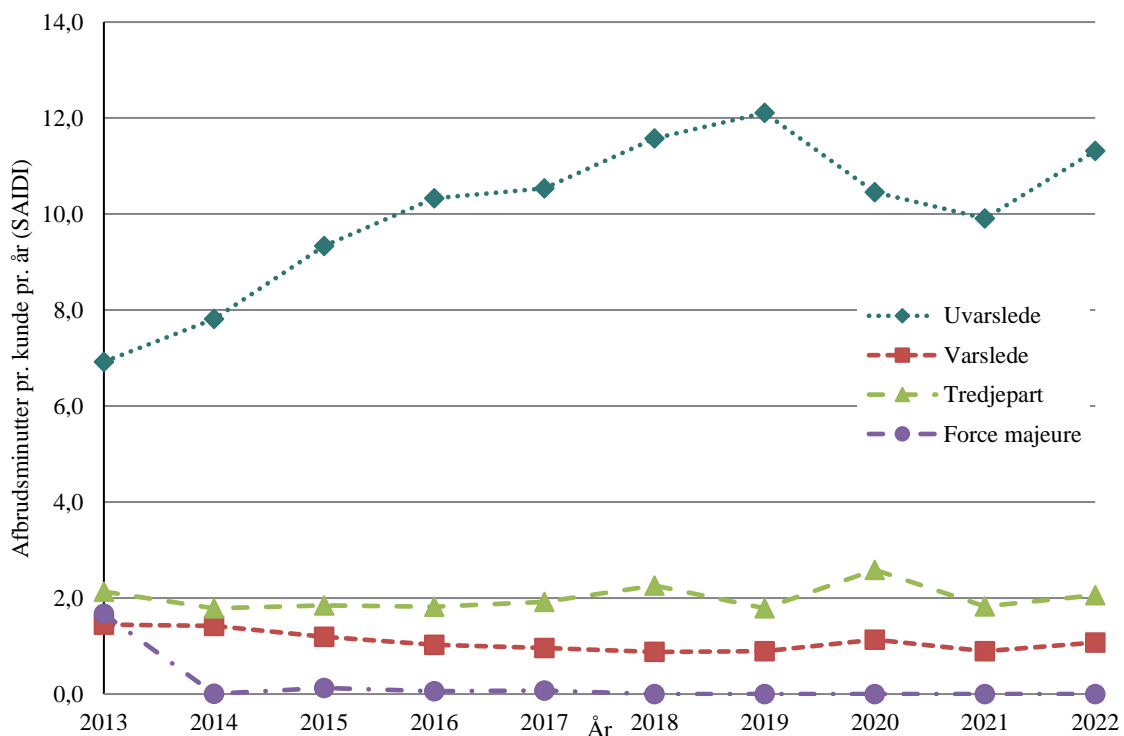
Figur 5.2 Gennemsnitlig kundefrafbrudsvarighed i minutter opgjort på 1-24-kV-statistikområdet (SAIDI)
