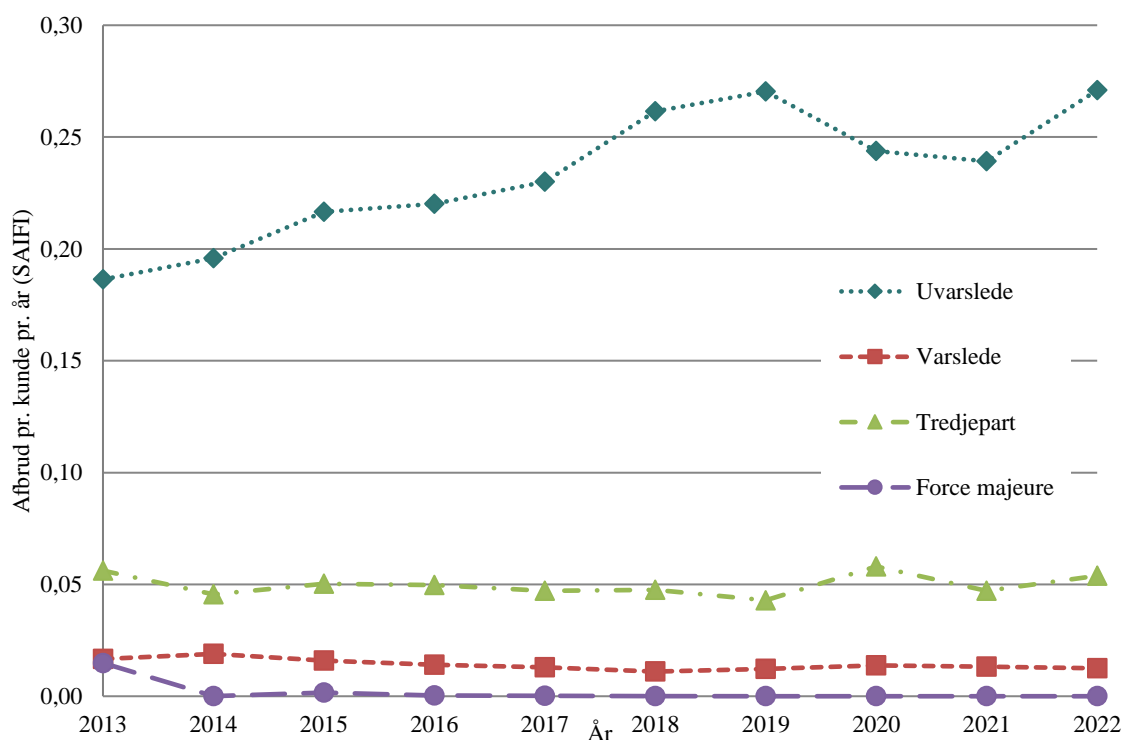
Figur 5.4 Gennemsnitlig kundeafbrudshyppighed opgjort på 1-24-kV-statistikområdet (SAIFI)
