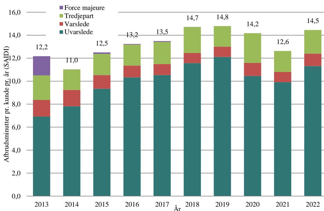
Figur 5.1 Fordelingen af den gennemsnitlige kundeforfbrudsvarighed i minutter opgjort på 1-24 kV-statistikområdet (SAIDI)
